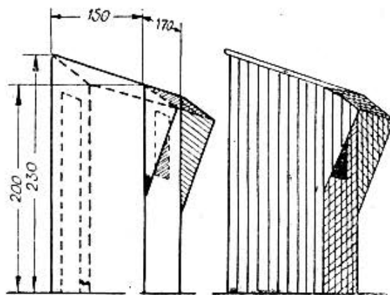
Rys. 60. Budka
