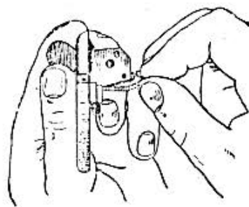
Rys. 40. Wyjmowanie zaczepu kurkowego
