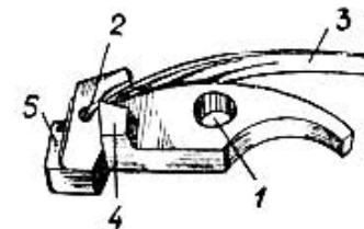
Rys. 23. Zaczep kurkowy:
