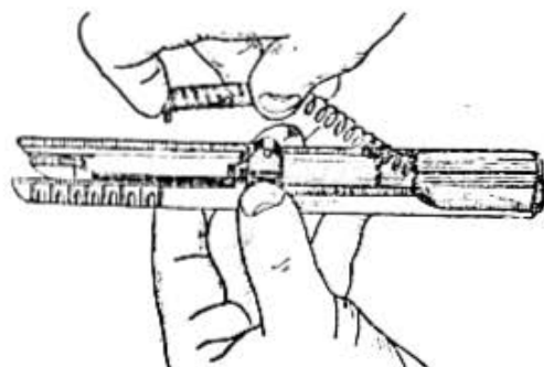
Rys. 36. Wyjmowanie sprężyny powrotnej
