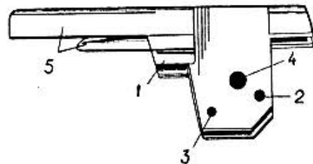
Rys. 20. Osada urządzenia spustowo-uderzeniowego:
