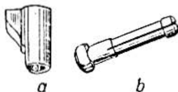
Rys. 17. Zatrask magazynka: a) tulejka; b) sworzeń
