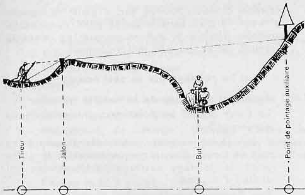
Pointage par un seul homme Point de pointage auxiliaire derrière le but
