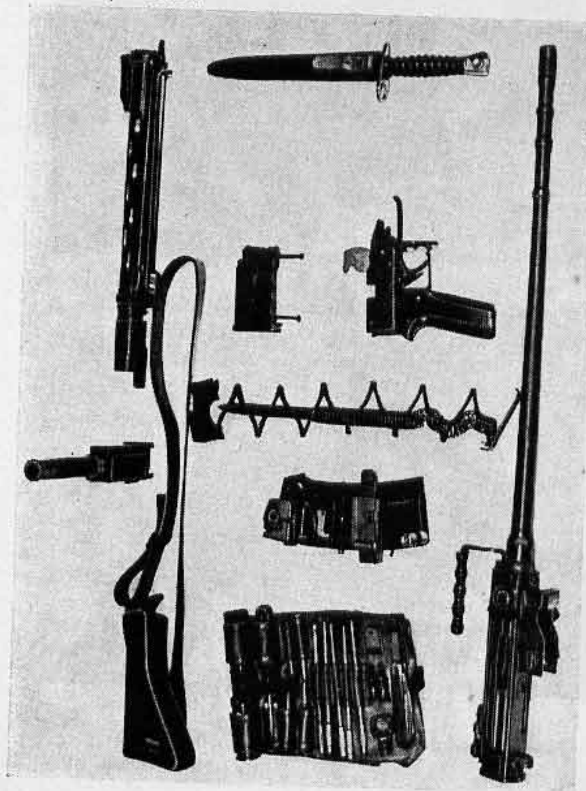
fig 24 Grand démontage (Disposition possible après le démontage)
