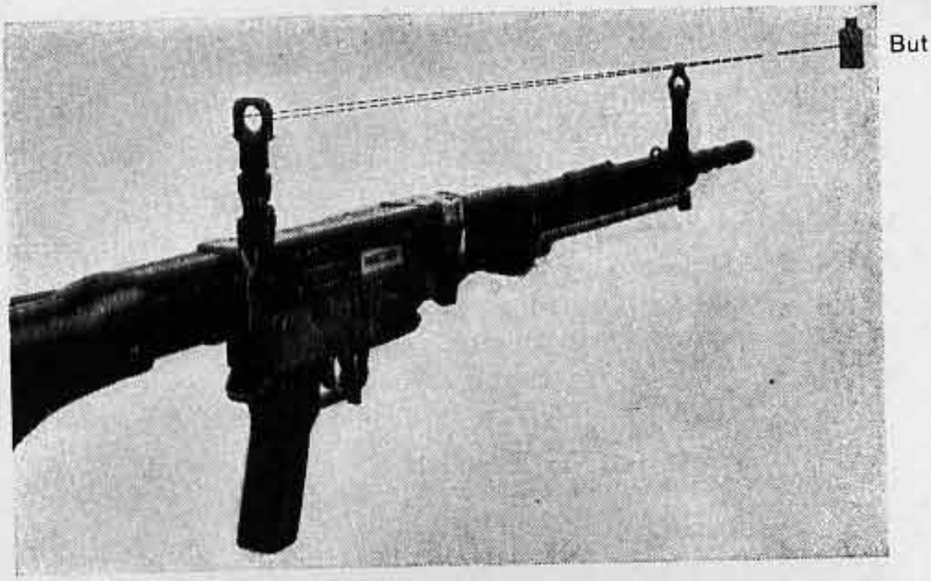
fig 47 Visée avec le dispositif de visée pour tir nocturne
