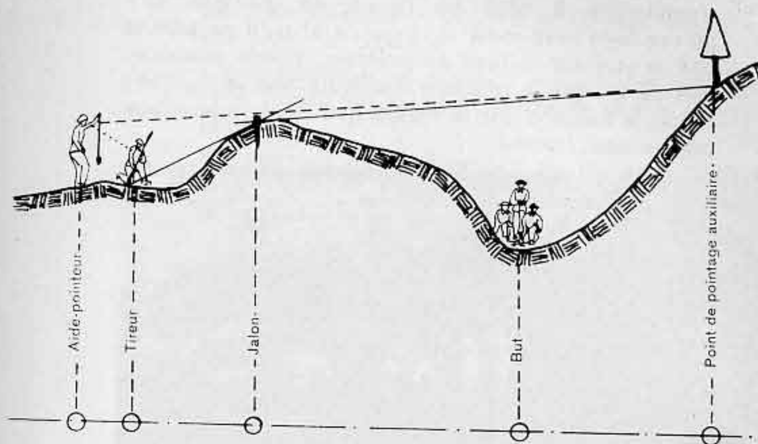
Pointage par deux hommes Point de pointage auxiliaire dans la zone des positions
