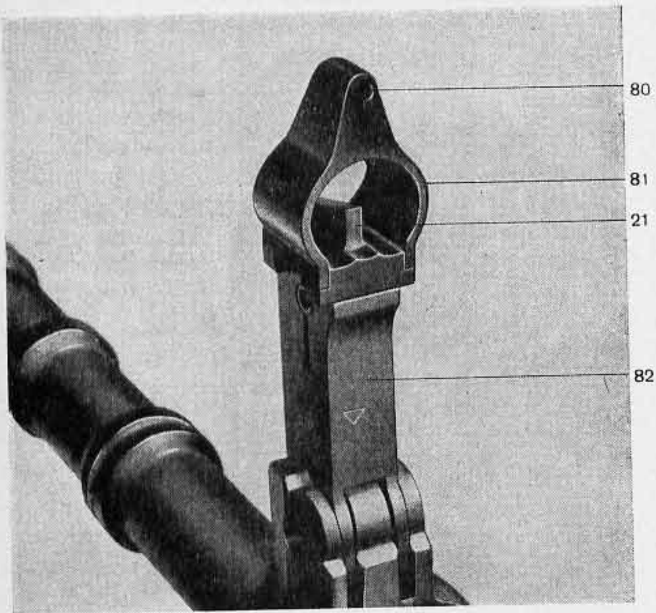
fig 9 Dispositif de visée : guidon
