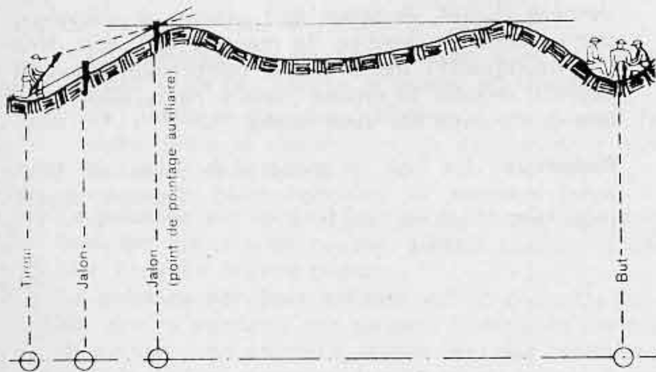
Pointage par un seul homme Point de pointage auxiliaire dans la zone des positions
