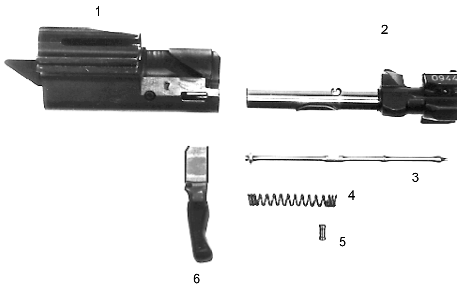
Figure 4: Culasse démontée
