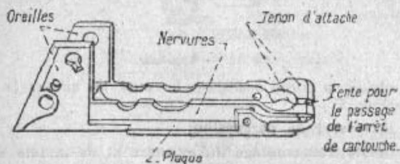
Fig. 14. — Corps de mécanisme de répétition.
