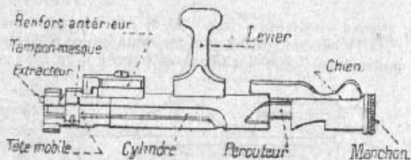
Fig. 6. — Culasse mobile.
