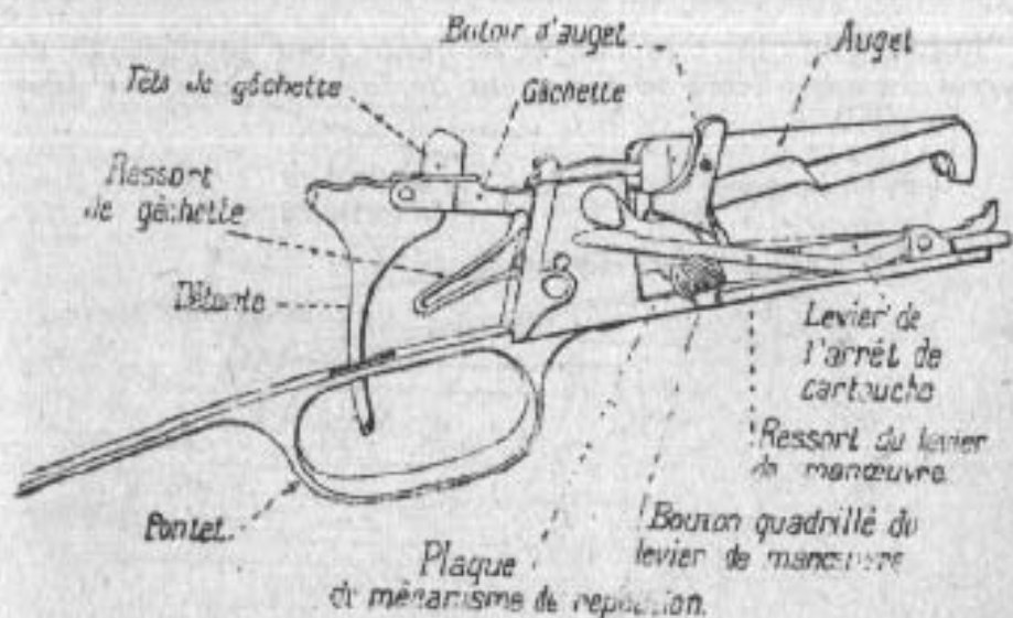
Fig. 13. — Mécanismes.
