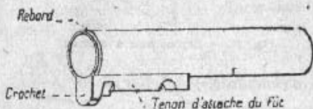
Fig. 22. — Tube-arrêt de piston.
