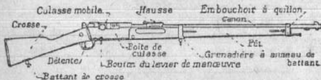
Fusil 86-93.
