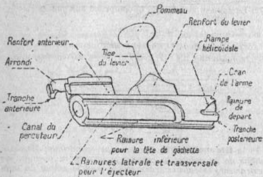
Fig. 9. — Cylindre.
