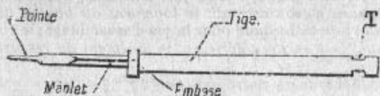
Fig. 11. — Percuteur.
