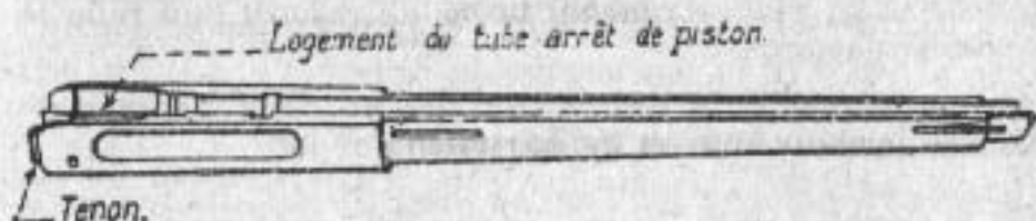
Fig. 21. — Fût.
