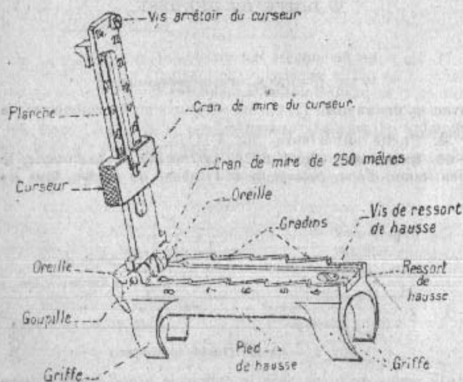
Fig. 3. — Hausse.
