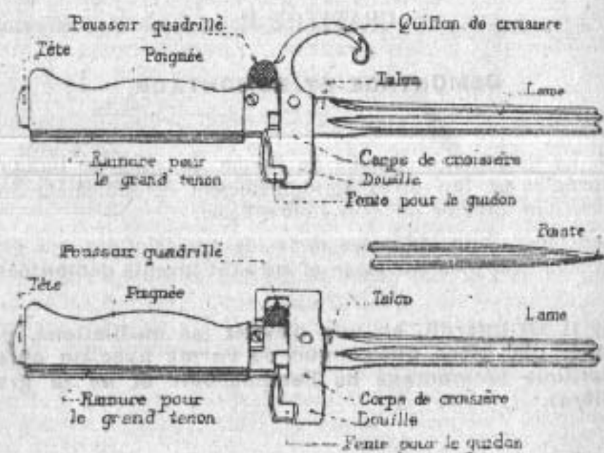
Fig. 27. — Épée-baïonnette.
