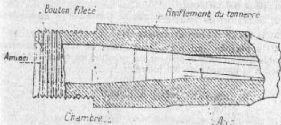
Fig. 1. — Canon. (Partie postérieure.)
