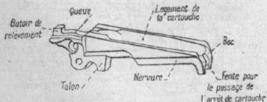
Fig. 15. — Auget.
