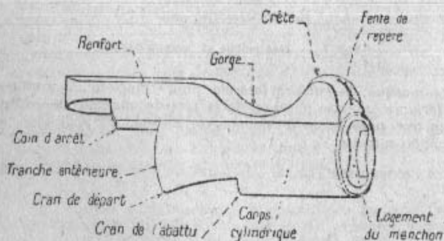
Fig. 10. — Chien.
