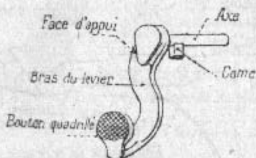
Fig. 17. — Levier de manœuvre.
